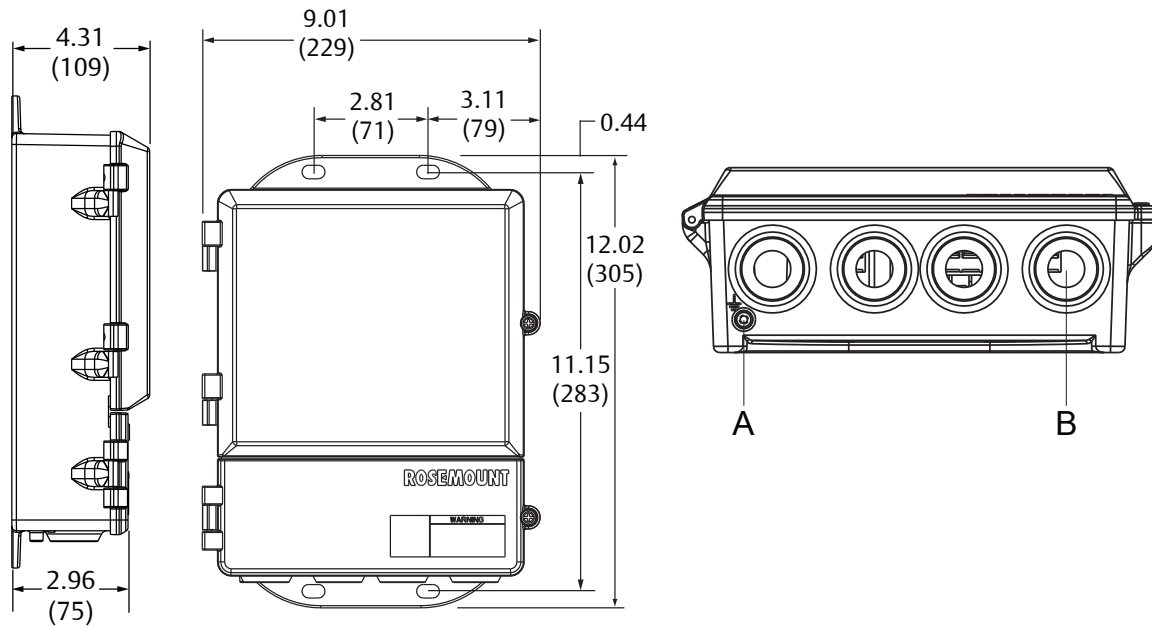
图 8: 带标准盖的墙装型变送器
