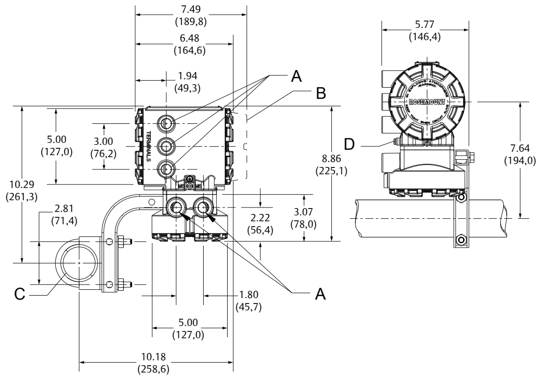
图 6: 分体式现场安装型变送器
