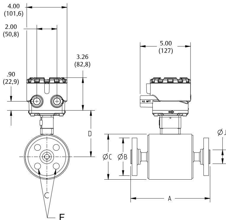
图 10: 凸面法兰型传感器, 1/2 英寸至 2 1/2 英寸 ( 15 毫米至 65 毫米 )
