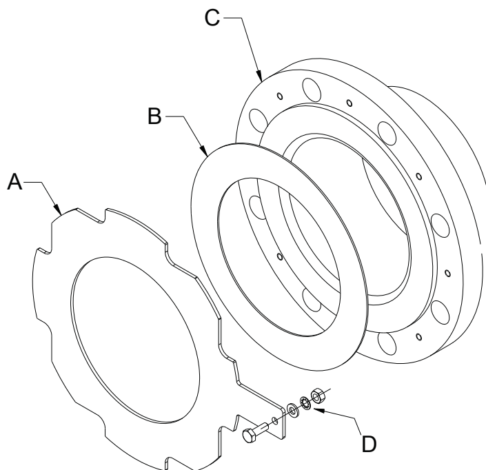
图 13: 法兰型传感器 ½ 英寸至 48 英寸 ( 15 毫米至 1200 毫米 ) 接地环
