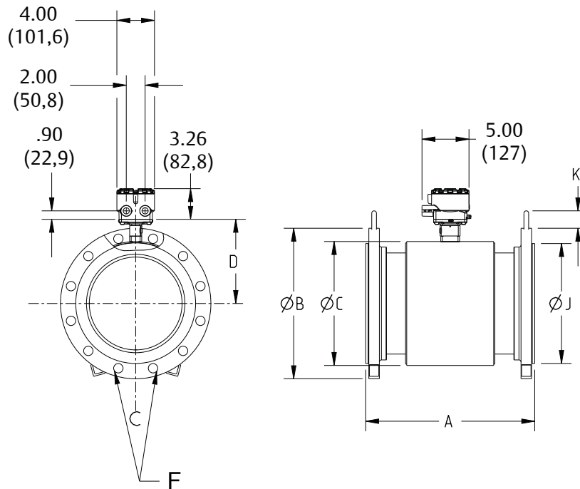
图 11: 凸面法兰型传感器, 3 英寸至 48 英寸 ( 75 毫米至 1200 毫米 )
